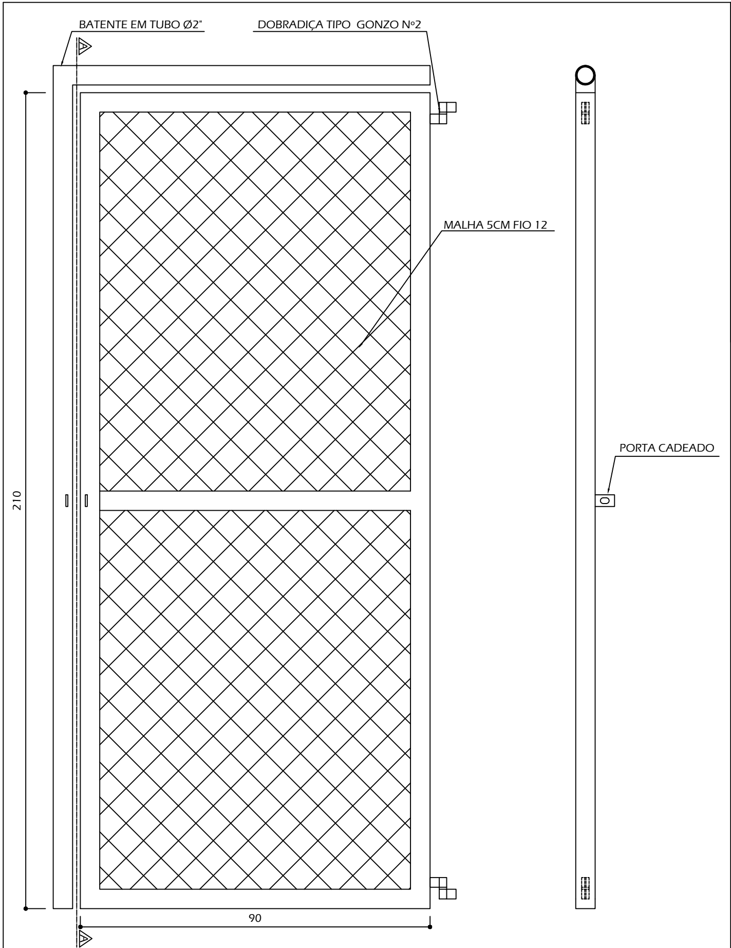
PORTÃO DE ALAMEDADO - ELEVACÃO
