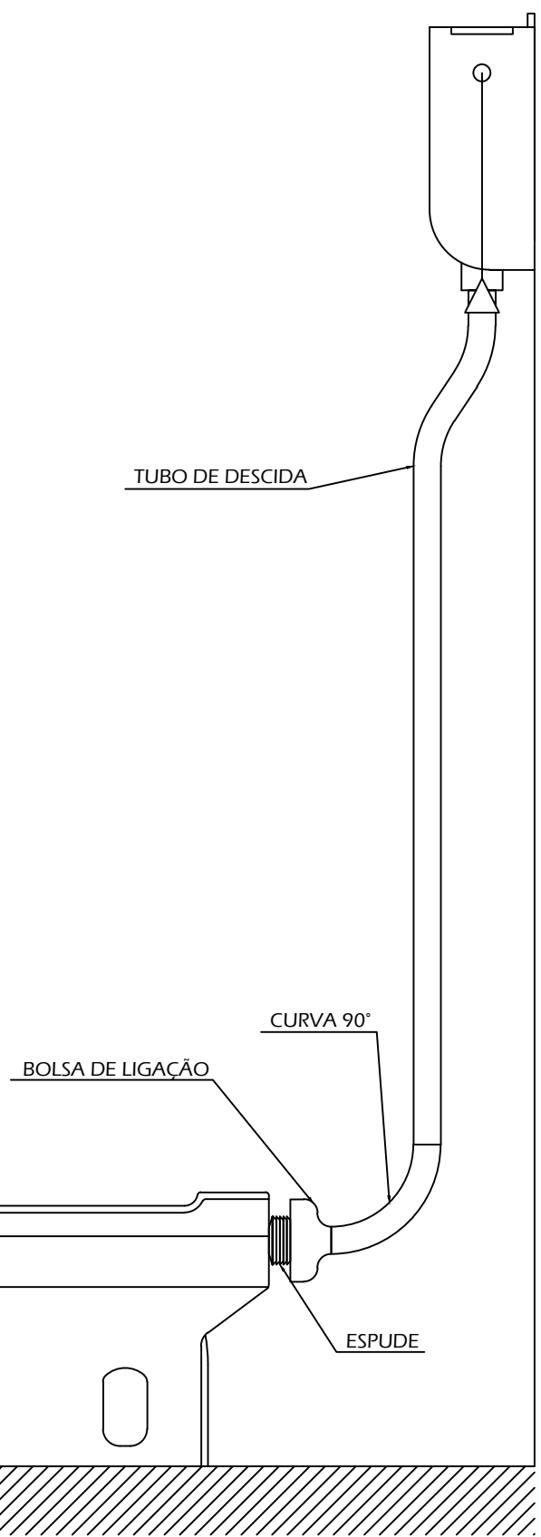
VISTA LATERAL - INSTALAÇÃO
