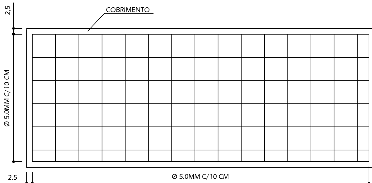
DETALHE 1 - ARMAÇÃO LONGITUDINAL E TRANSVERSAL DA BANCADA
