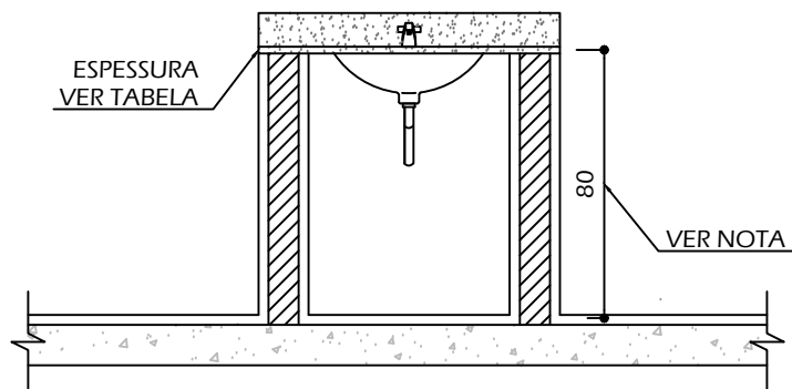
ELEVAÇÃO A - BANCADA DE LAVATÓRIO
