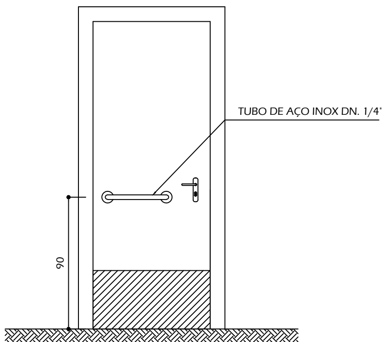
ELEVAÇÃO - BARRA INSTALADA EM PORTA
