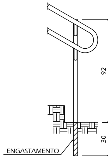
ELEVAÇÃO - PARTE INFERIOR ESCALA 1/20
