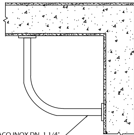
VISTA EM PLANTA - BARRA DE CANTO
