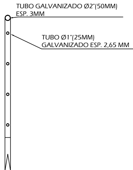
CORTE D-D ESCALA 1/20
