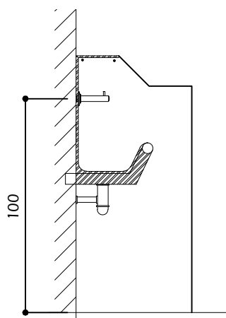
TIPO 13 - TORNEIRA BEBEDOURO DE PAREDE C/ FECHAMENTO AUTOMÁTICO
