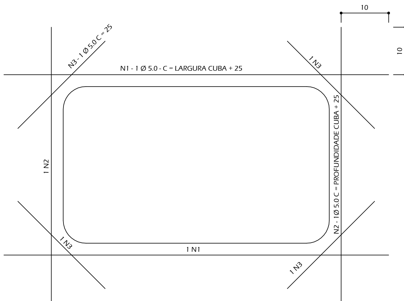
DETALHE 2 - ARMAÇÃO DO FURO PARA BOJO
