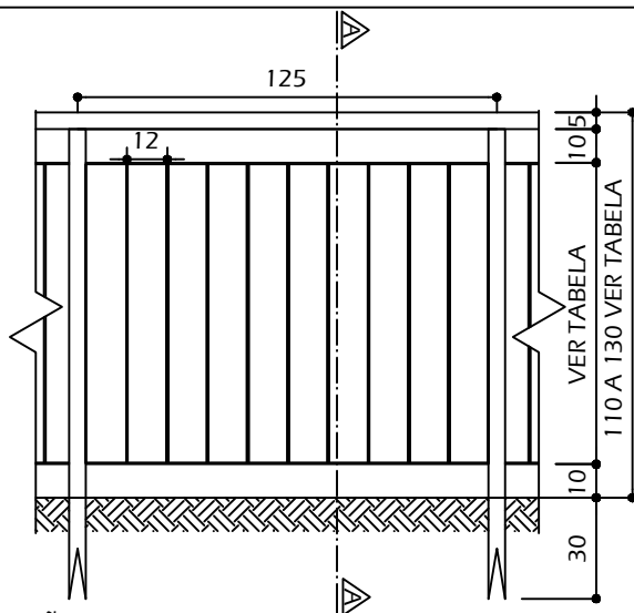
ELEVÇÃO
