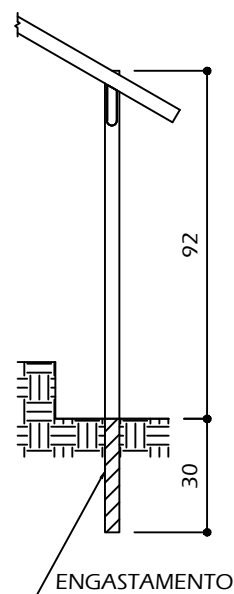
ELEVAÇÃO - PARTE INFERIOR ESCALA 1/20
