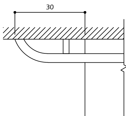
PLANTA - PARTE SUPERIOR ESCALA 1/10
