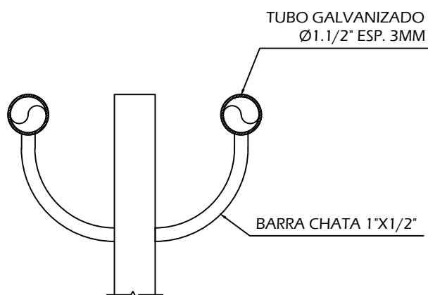
CORTE E-E
