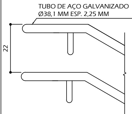
ELEVAÇÃO - PARTE SUPERIOR
