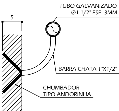
CORTE A-A ESCALA 1/5
