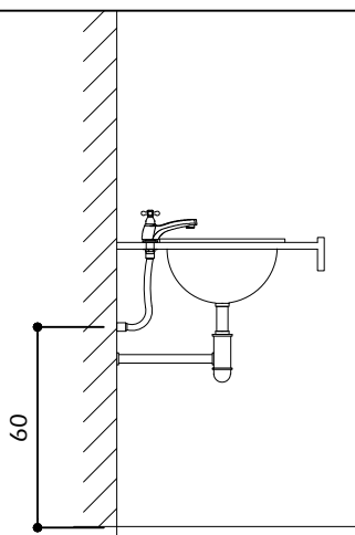
TIPO 1 - TORNEIRA LAVATÓRIO DE MESA C/ AREJADOR
