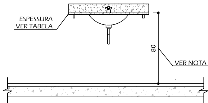
ELEVAÇÃO A - BANCADA DE LAVATÓRIO
