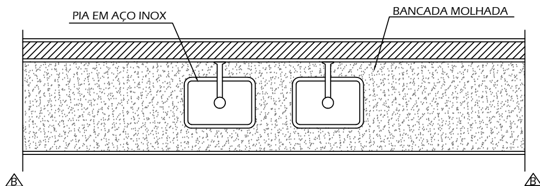
PLANTA - BANCADA DE PIA
