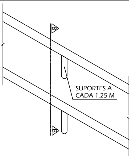
ELEVAÇÃO - MEIO
