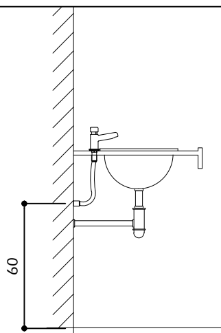
TIPO 2 - TORNEIRA LAVATÓRIO DE MESA C/ FECHAMENTO AUTOMÁTICO
