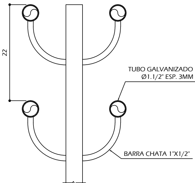
CORTE F-F ESCALA 1/10
