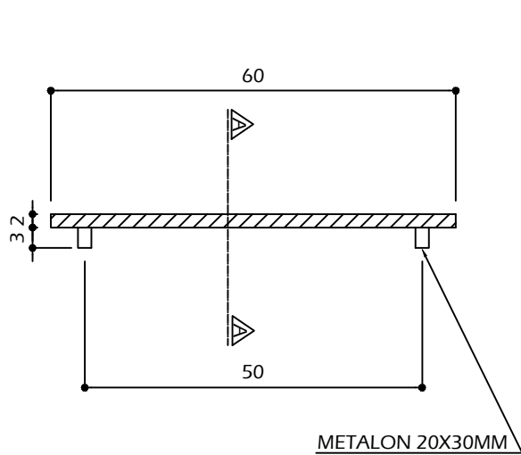
VISTA - PRATELEIRA SOBRE METALON ESCALA 1/10
