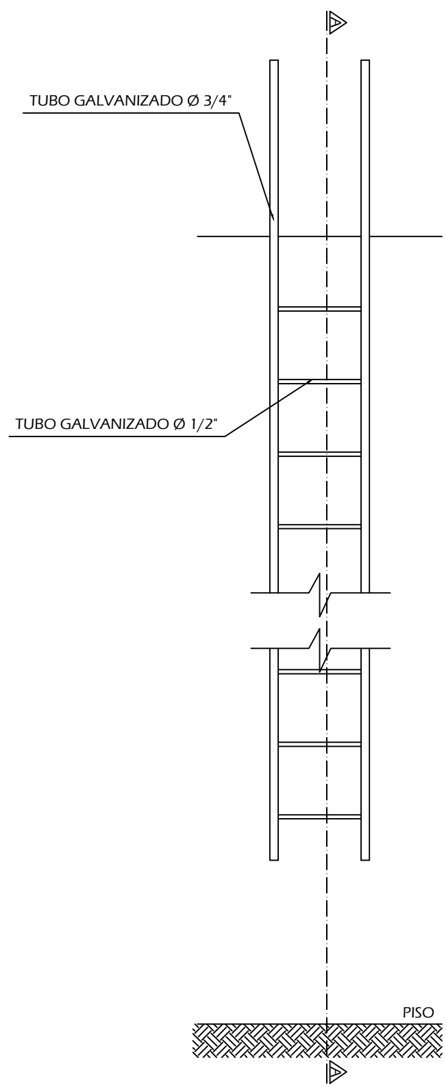
VISTA FRONTAL ESCALA 1/25
