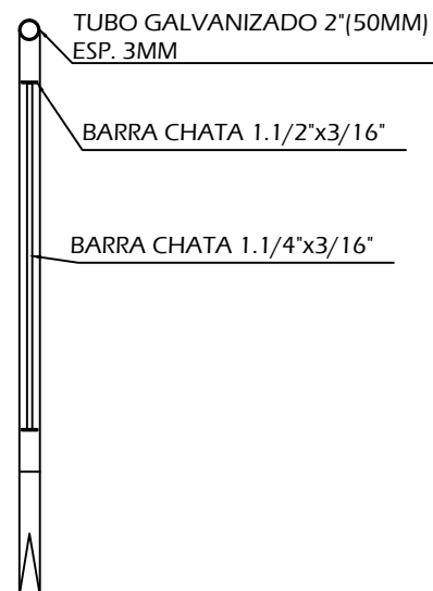
CORTE A-A
