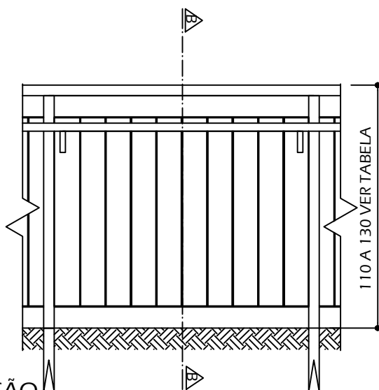
ELEVÇÃO
