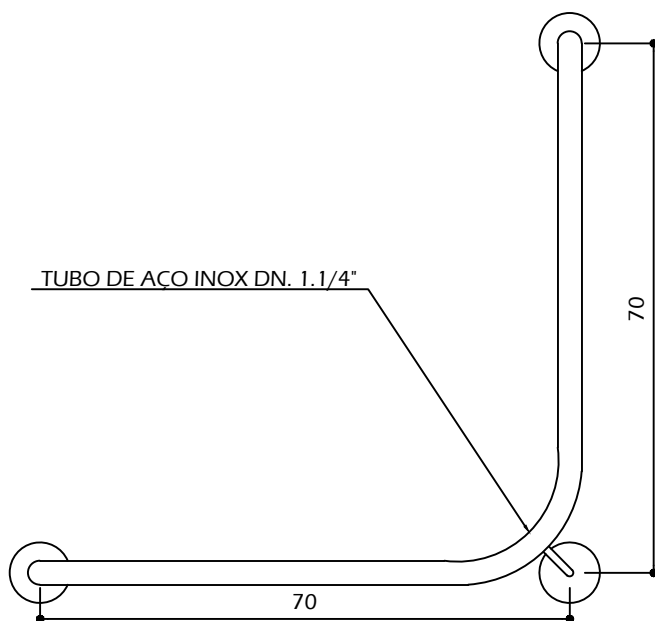
VISTA LATERAL - BARRA L
