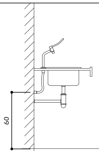
TIPO 3 - TORNEIRA HOSPITALAR DE MESA ALAVANCA COTOVELO 1/4 VOLTA
