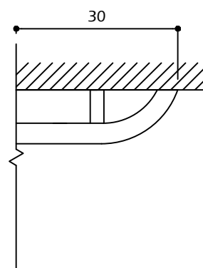
PLANTA - PARTE INFERIOR ESCALA 1/10
