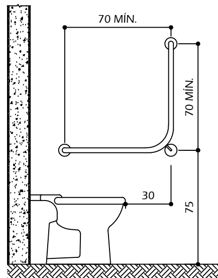
ELEVAÇÃO - BARRA L INSTALADA EM SANITÁRIO
