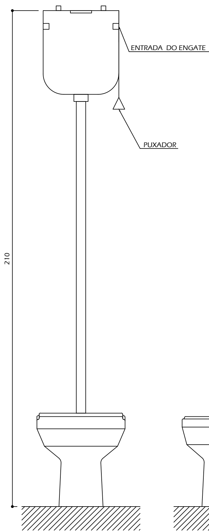
VISTA FRONTAL - INSTALAÇÃO
