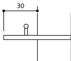
ELEVAÇÃO - PARTE SUPERIOR ESCALA 1/20
