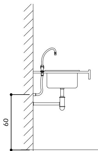
TIPO 4 - TORNEIRA PIA BICA ALTA MÓVEL DE MESA
