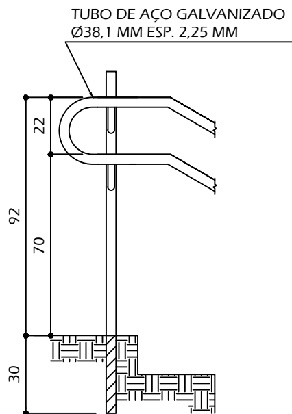
ELEVAÇÃO - PARTE SUPERIOR ESCALA 1/20
