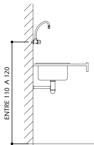
TIPO 6 - TORNEIRA PIA BICA ALTA MÓVEL DE PAREDE
