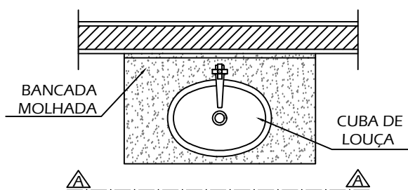
PLANTA - BANCADA DE LAVATÓRIO
