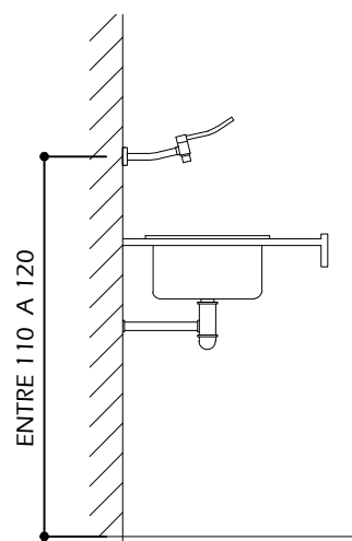
TIPO 5 - TORNEIRA HOSPITALAR DE PAREDE ALAVANCA COTOVELO 1/4 VOLTA
