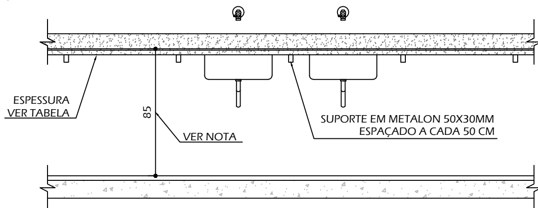
PLANTA - BANCADA DE PIA
