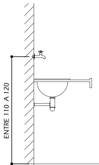
TIPO 8 - TORNEIRA GERAL DE PAREDE
