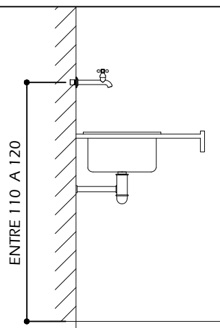
TIPO 11 - TORNEIRA PIA LONGA DE PAREDE
