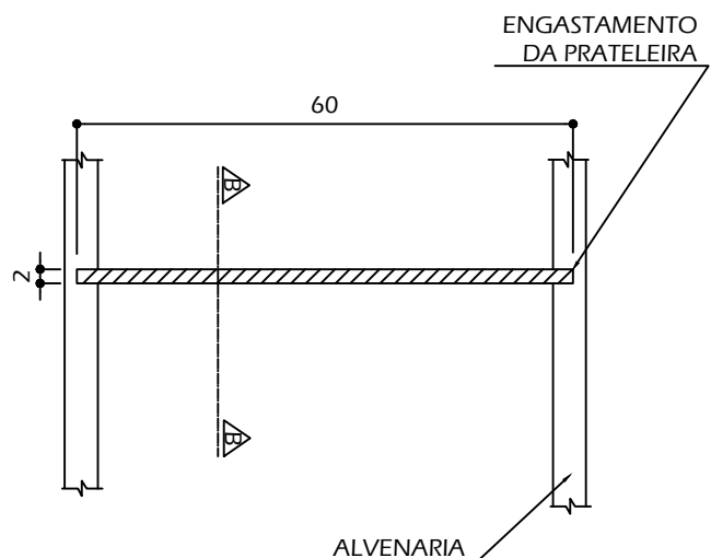
VISTA - PRATELEIRA ENTRE ALVENARIAS ESCALA 1/10
