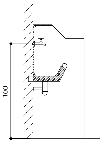
TIPO 12 - TORNEIRA BEBEDOURO/ TANQUE DE PAREDE BICO LISO
