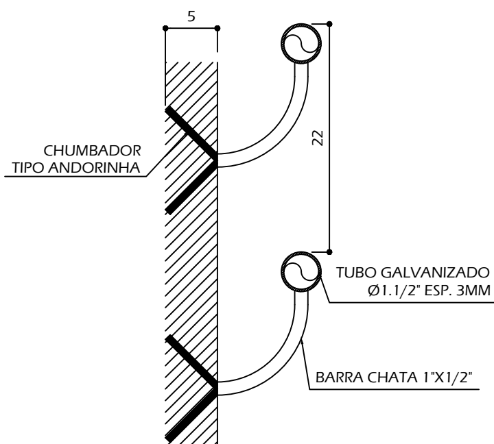
CORTE B-B
