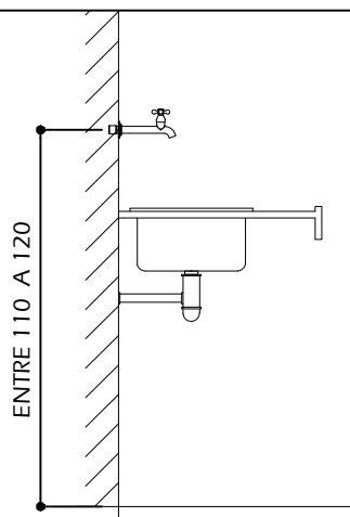
TIPO 10 - TORNEIRA PIA LONGA DE PAREDE C/ BICO LISO
